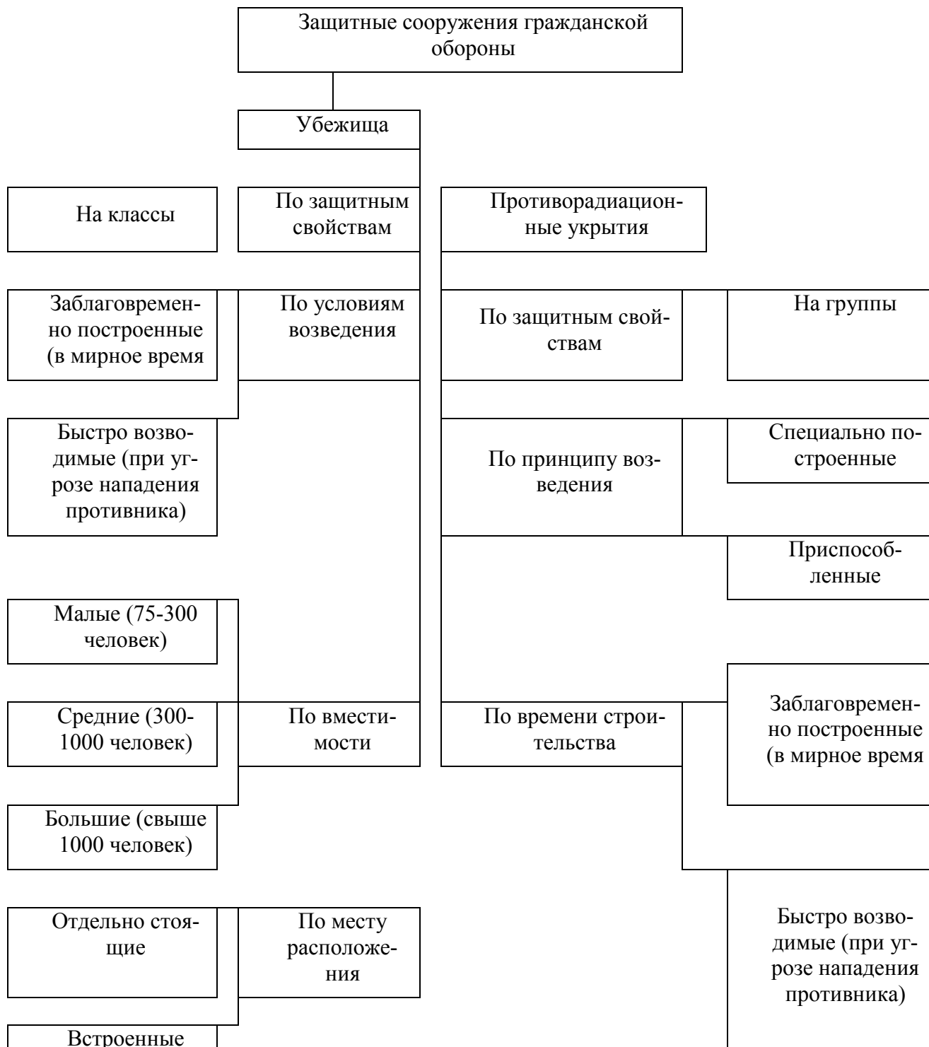
Классификация коллективных средств защиты
