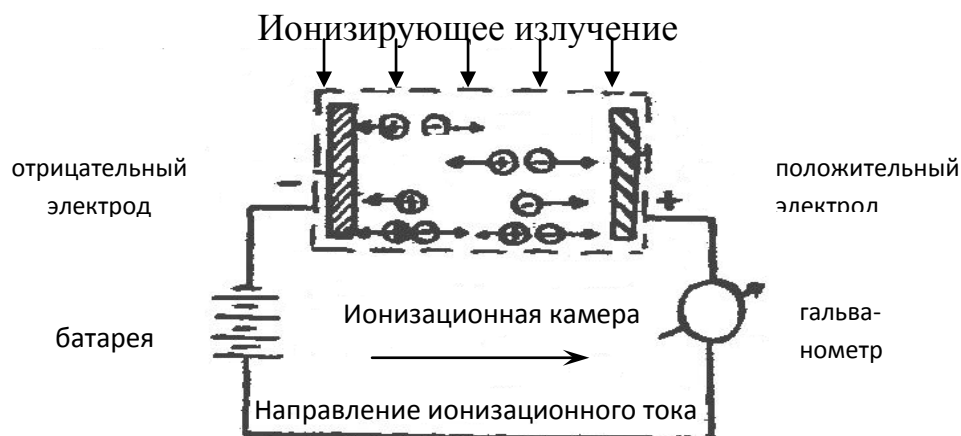
Рис. 1 Принцип работы ионизационной камеры
